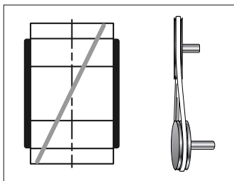
图5 显示垂直方向的角度不对中
