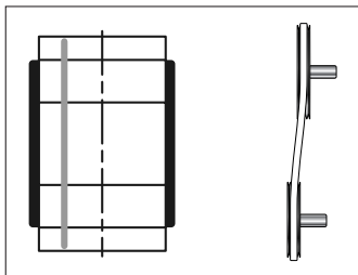
图7 显示平行不对中
